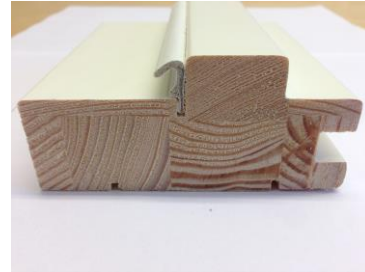
Snitt av karmside m/dempelist
